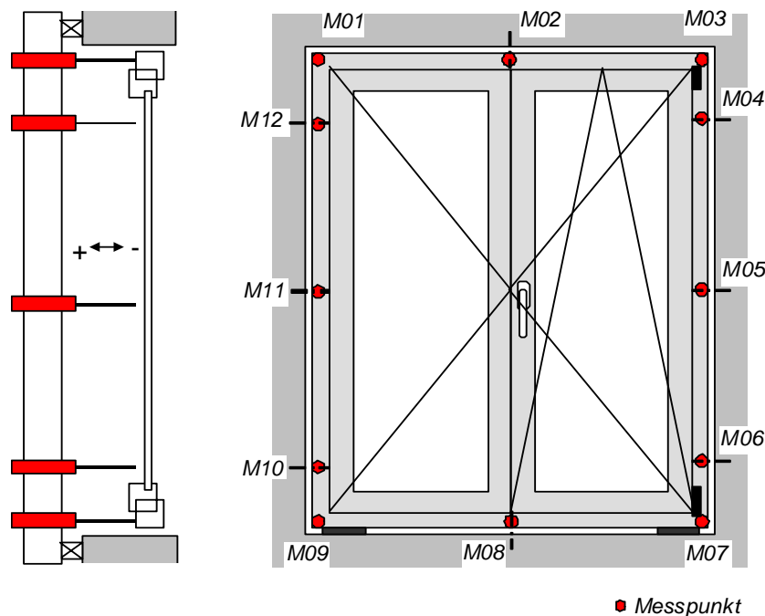
Bild 3 Schematische Darstellung der Position der Befestigungspunkte und der Linearpotentiometer
