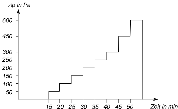
Abbildung 1 Darstellung der Druckstufen und des zeitlichen Verlaufes
