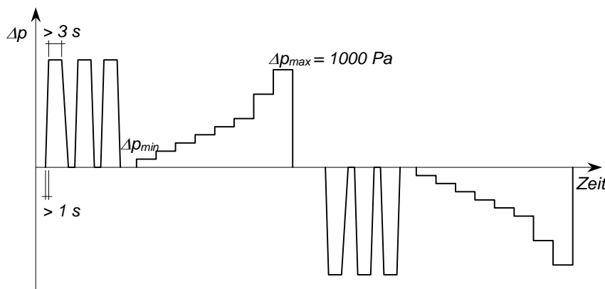
Abbildung 2 Prüfung Luftdurchlässigkeit bei Über- und Unterdruck
