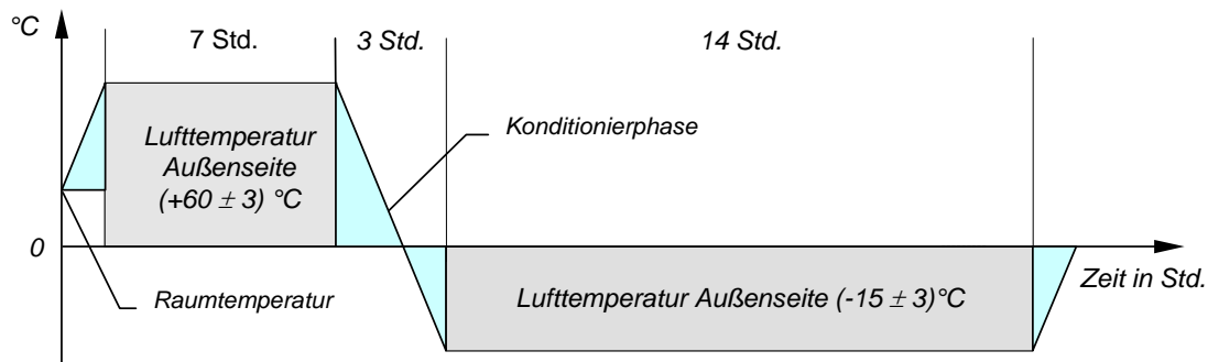
Abbildung 3 Darstellung der Temperatur-Wechselbelastung für einen Zyklus
